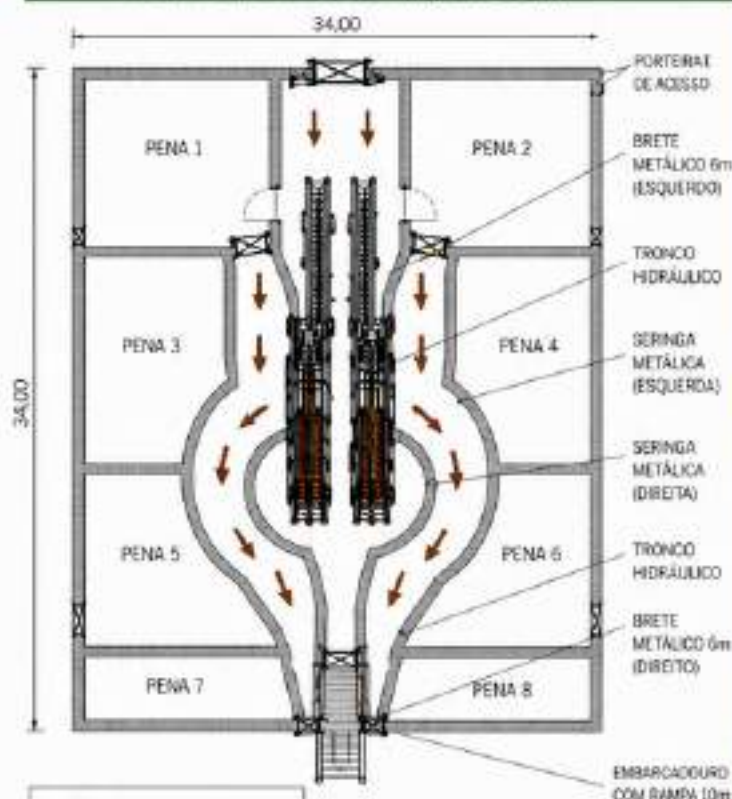
PLANTA BAIXA — 34 x 34 m (Brete Duplo)
