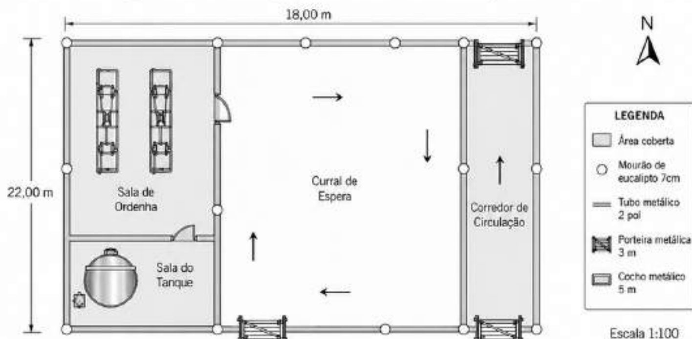
Planta Baixa — Ordenha Média — 18 x 22 m
