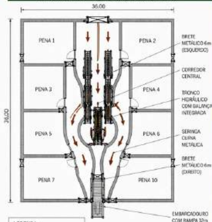
PLANTA BAIXA — 36 x 36 m (Layout Técnico)
