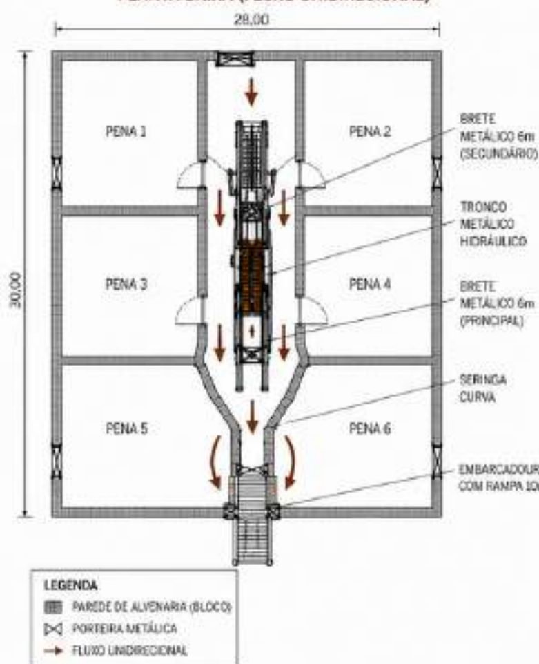
PLANTA BAIXA (FLUXO UNIDIRECIONAL)
