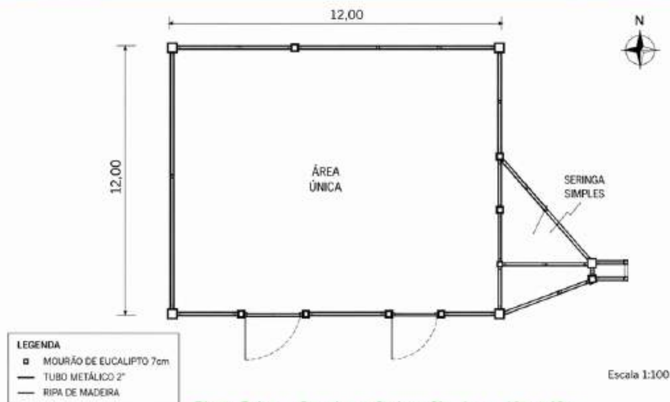
Planta Baixa — Curral com Seringa Simples — 12m x 12m
