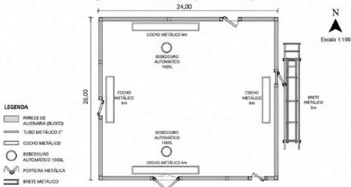
Planta Baixa — Curral Médio Estruturado — 24m x 26m
