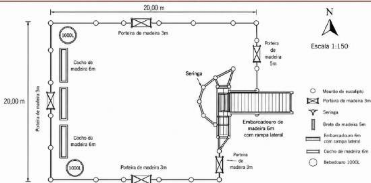
Planta Baixa — Curral Econômico 12 — 20x20m
