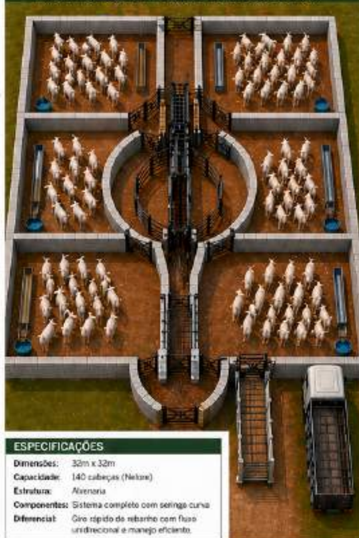
IMAGEM 3D ILUSTRATIVA (VISTA AÉREA ISOMÉTRICA)
