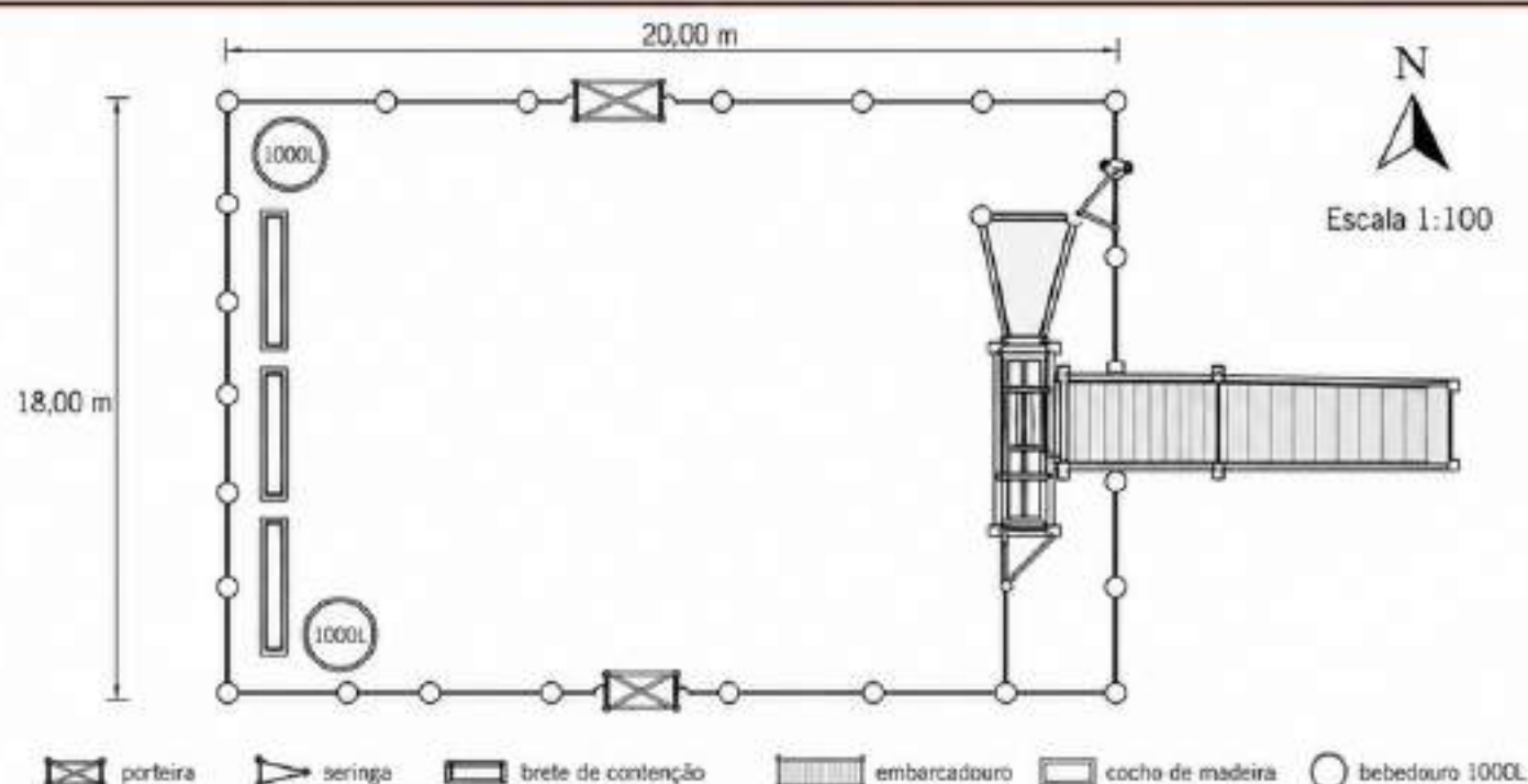
Planta Baixa — Curral Econômico 11 — 18x20m
