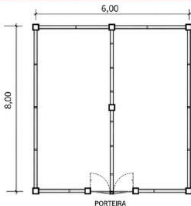
Planta Baixa — Curral Pequeno Rural — 6m x 8m
