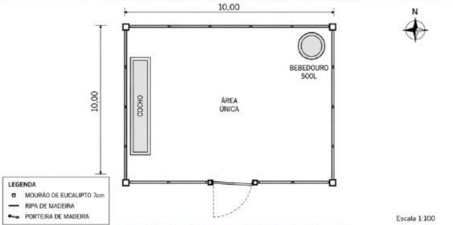
Planta Baixa — Curral Pequeno Funcional — 10m x 10m
