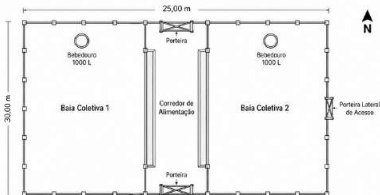
Planta Baixa — Confinamento Simples — 25 x 30 m
