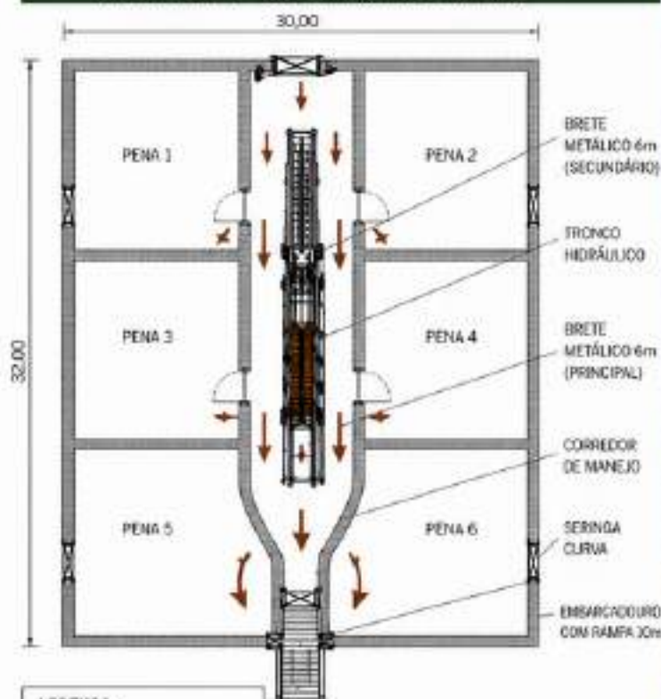
PLANTA BAIXA — 30 x 32 m (Fluxo Otimizado)
