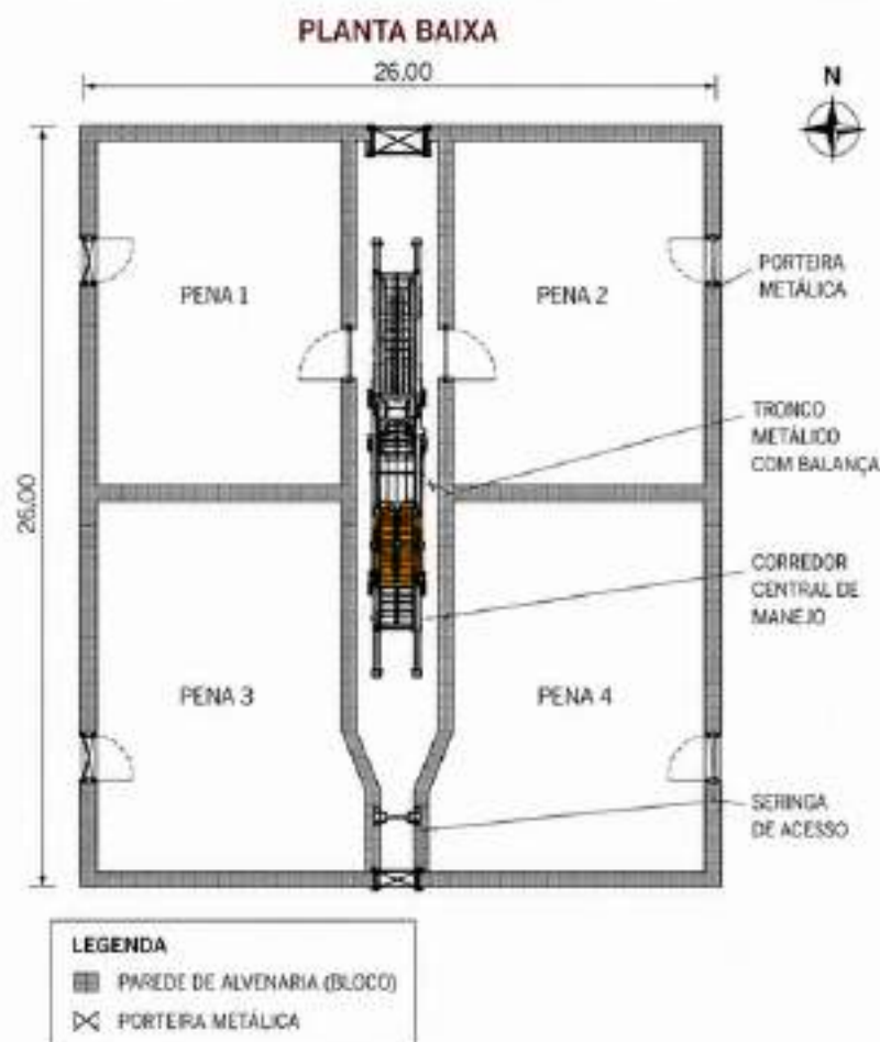
Planta Baixa — Curral Médio Profissional — 26m x 26m
