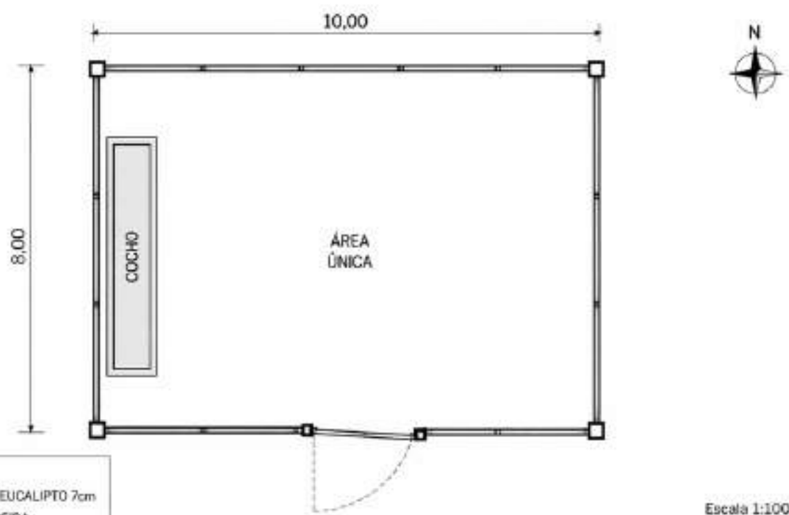
Planta Baixa — Curral Simples com Cocho — 8m x 10m
