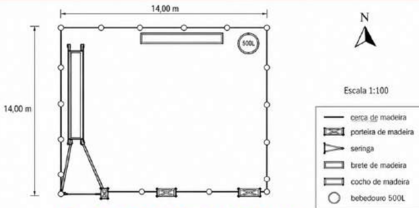
Planta Baixa — Curral Econômico 6 — 14 x 14 m
