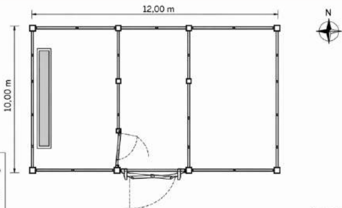
Planta Baixa — Curral Pequeno Reforçado — 10m x 12m
