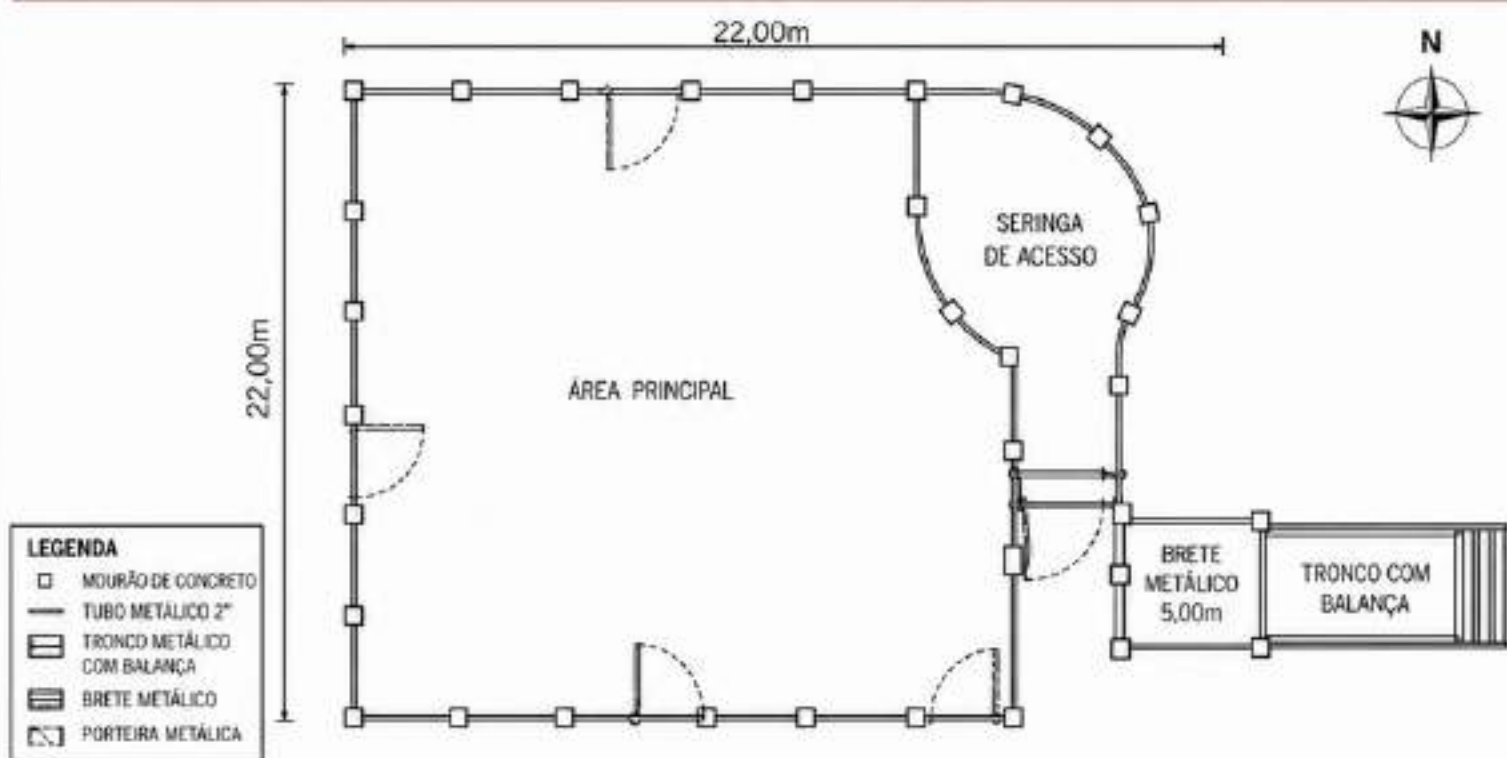
Planta Baixa — Curral Médio Técnico — 22m x 22m
