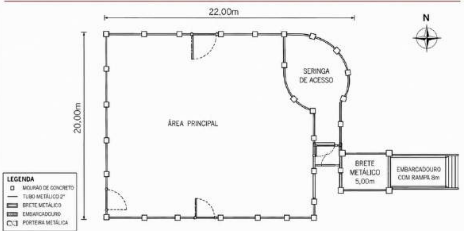
Planta Baixa — Curral Médio Operacional — 20m x 22m
