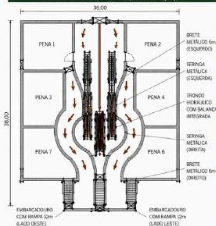
PLANTA BAIXA — 36 x 38 m (Sistema Duplo)
