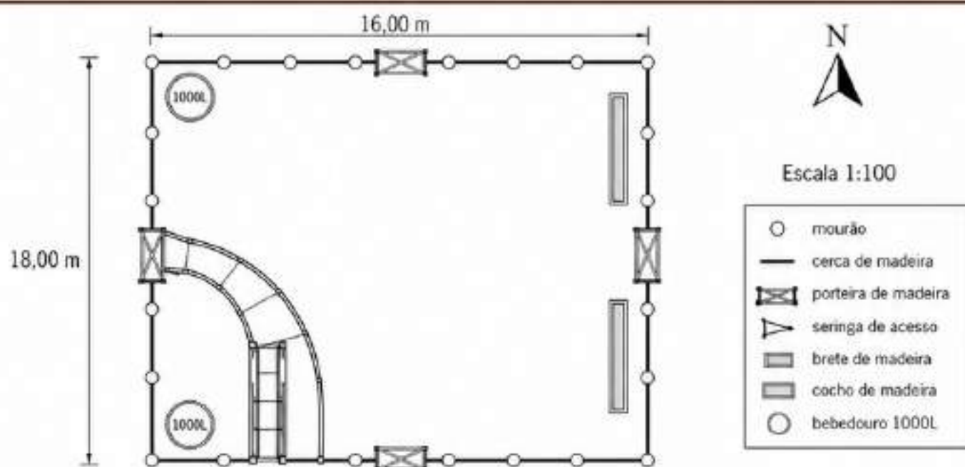
Planta Baixa — Curral Econômico 9 — 16x18m
