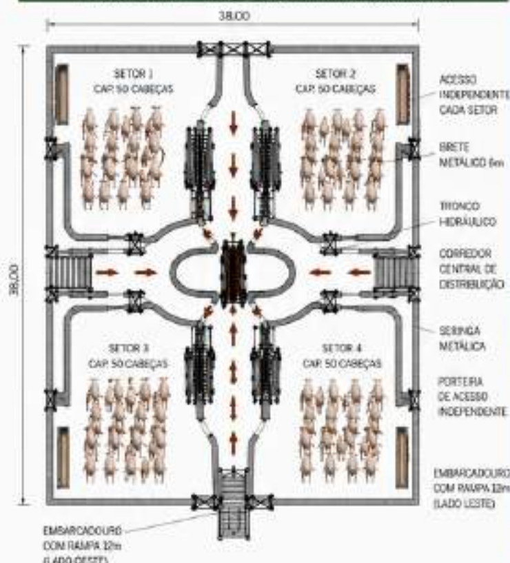
PLANTA BAIXA — 38 x 38 m (Setores Independentes)
