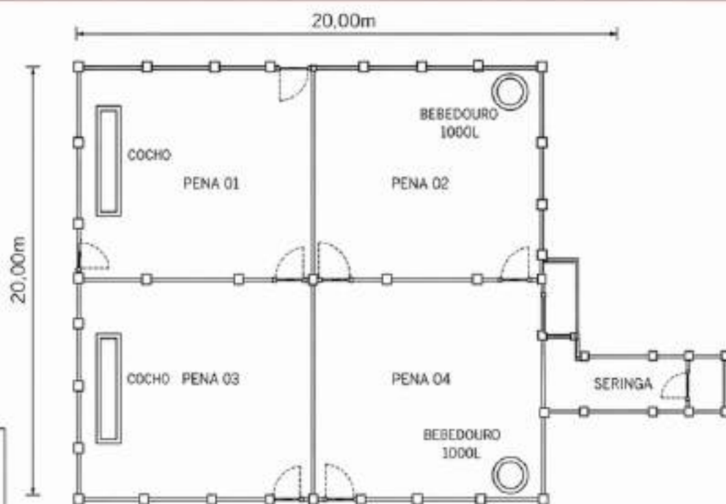
Planta Baixa — Curral Médio com Divisões — 20m x 20m
