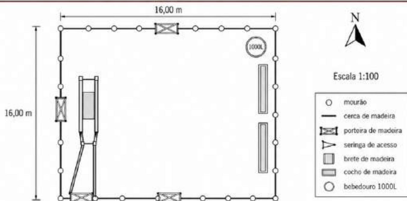
Planta Baixa — Curral Econômico 8 — 16x16m
