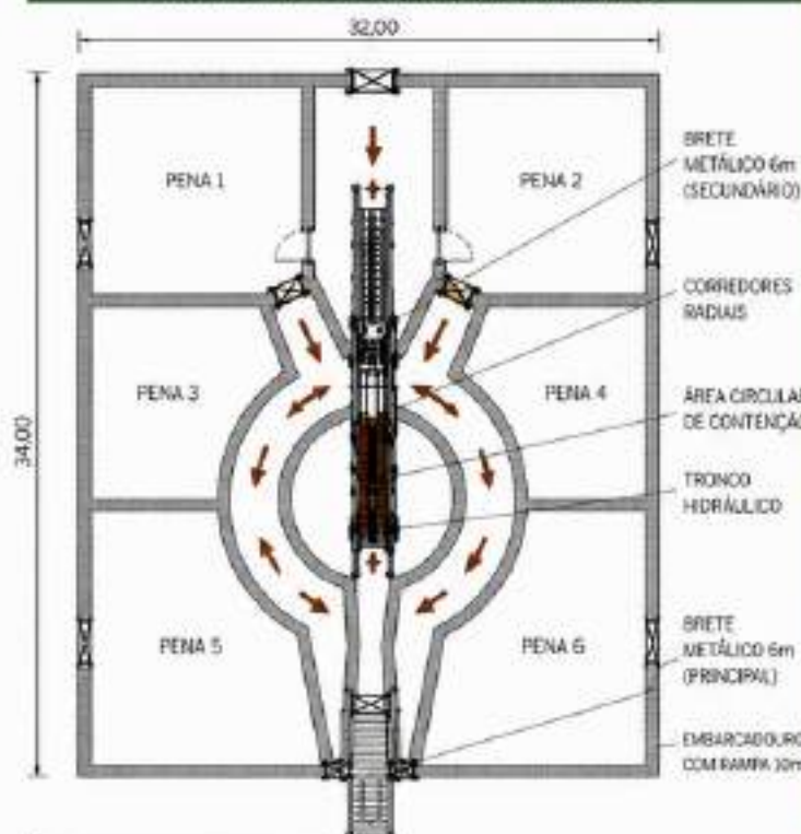
PLANTA BAIXA — 32 x 34 m (Fluxo Inteligente)
