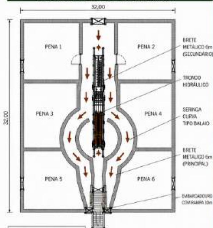
PLANTA BAIXA — 32 x 32 m (Fluxo de Manejo)
