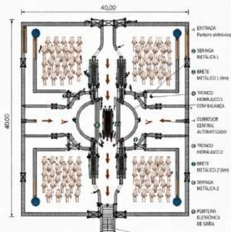
PLANTA BAIXA — 40 x 40 m (Automação Parcial)
