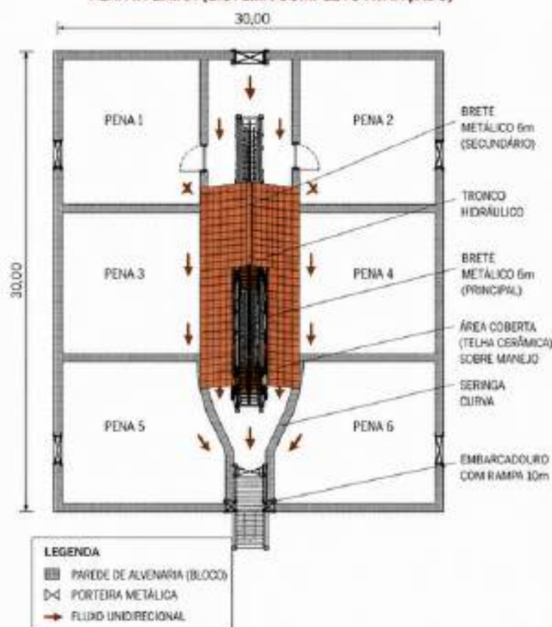
PLANTA BAIXA (SISTEMA COMPLETO AVANÇADO)
