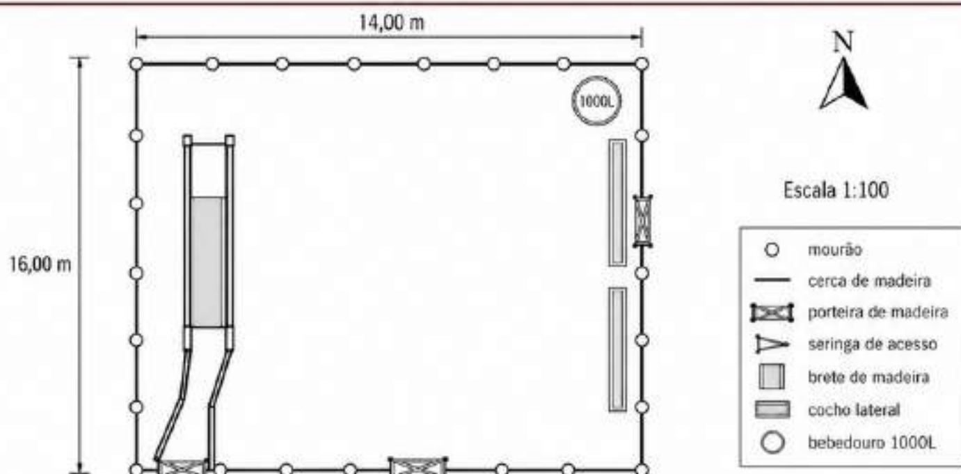
Planta Baixa — Curral Econômico 7 — 14x16m
